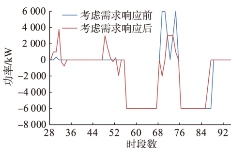
图7 需求响应前后储能功率变化
