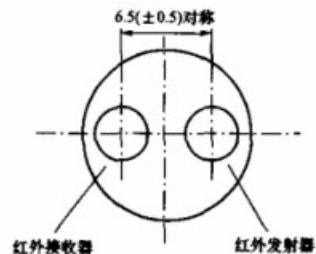
图 3 光口正视图
