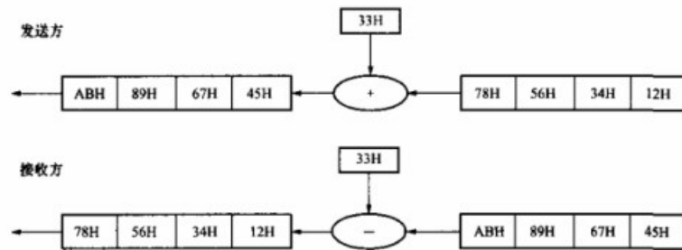
图9 传输次序图
