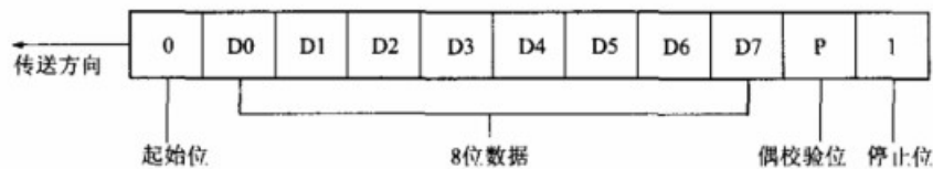
图 7 字节传输序列
