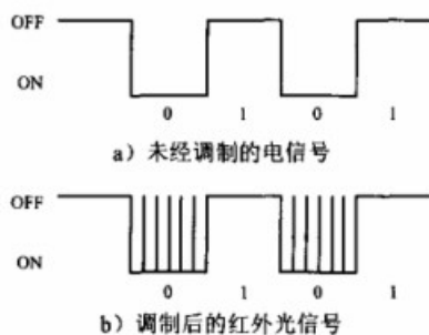
图5 信号与调制
