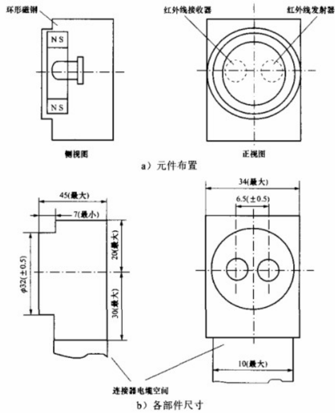
图 1 读数头的结构
