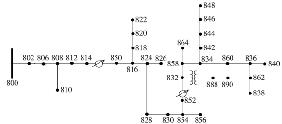
图 4 IEEE 34 节点配电系统单线图
