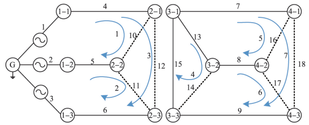
图 2 IEEE 4 节点标准配电网拓扑图
